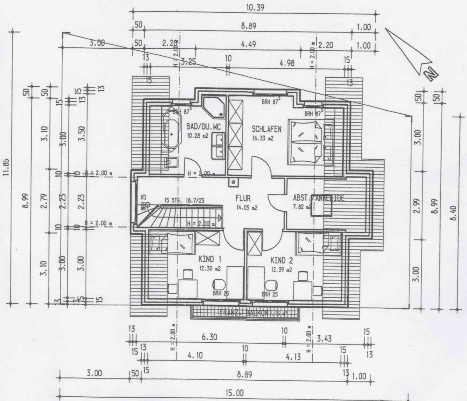
GRUNDRISS DACHGESCHOSS
