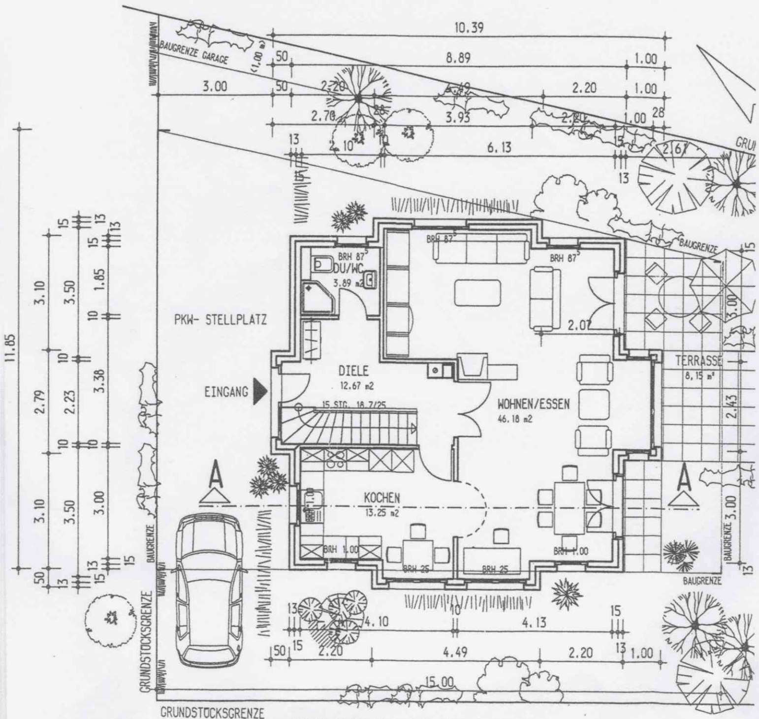
GRUNDRISS ERGESCHOSS
